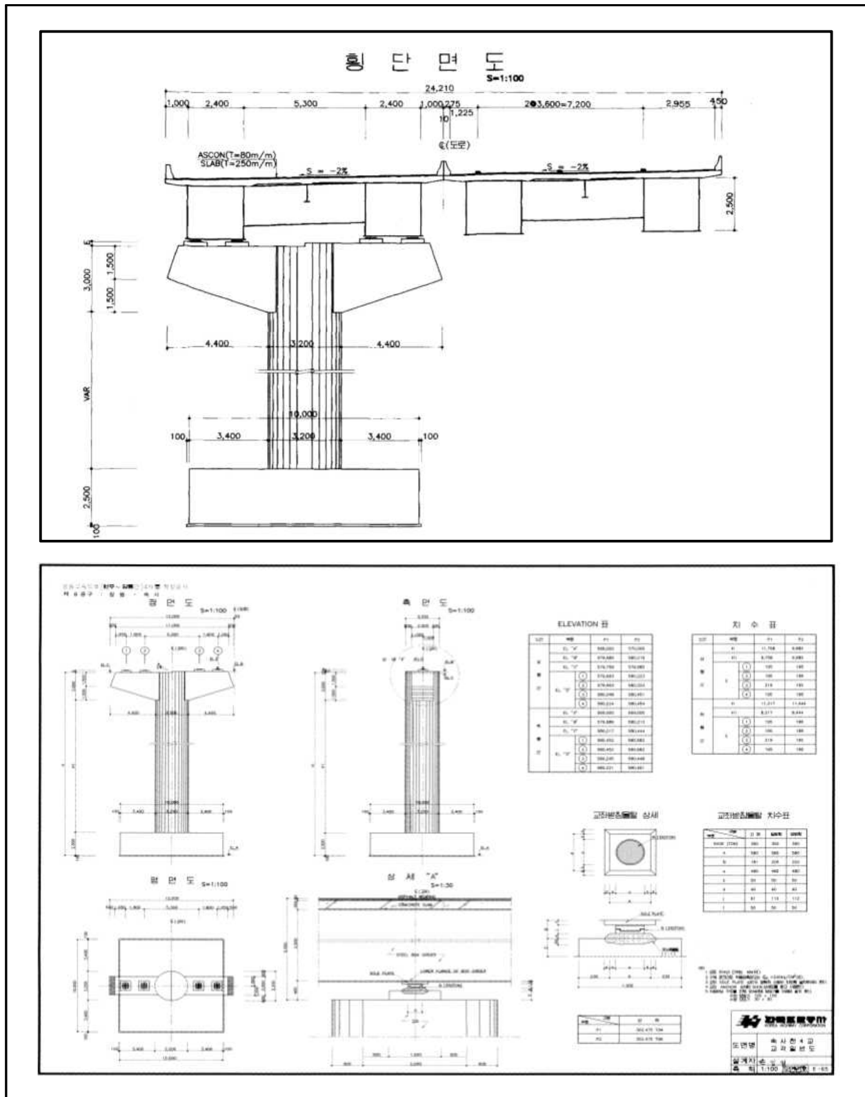
【그림 1.3】 교각 일반도
