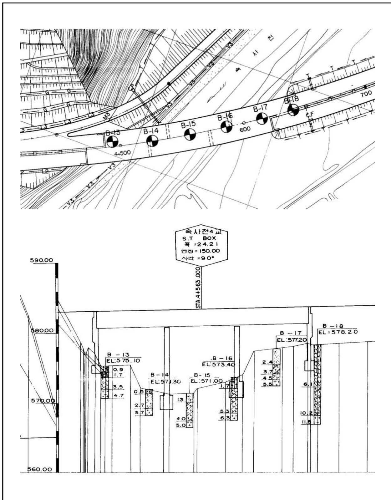
【그림 1.2】 종·평면도
